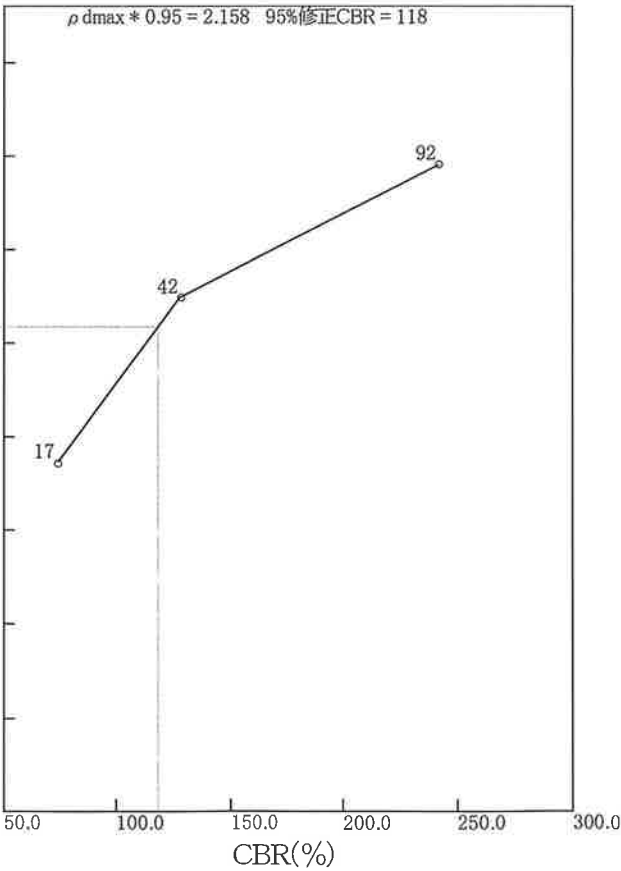
乾燥密度－CBR曲線
