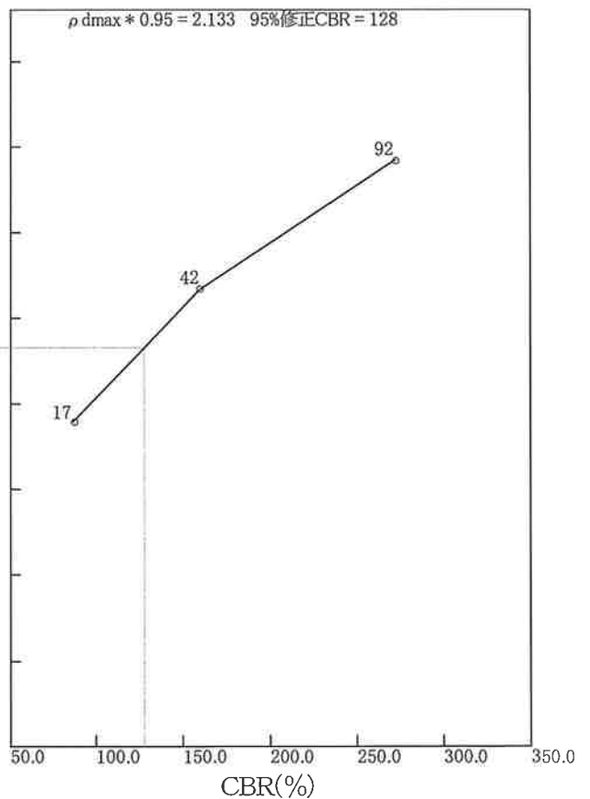
乾燥密度－CBR曲線
