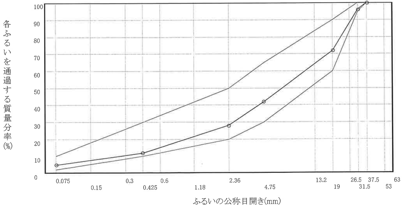
粒度曲線
