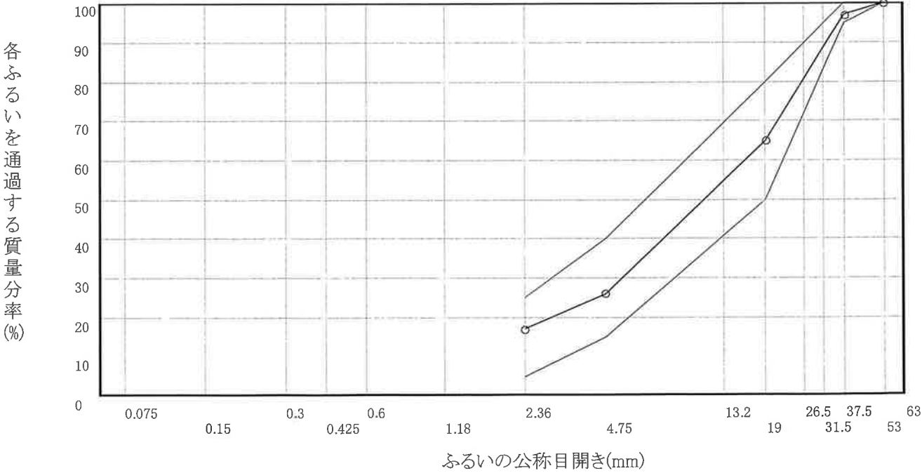
粒度曲線
