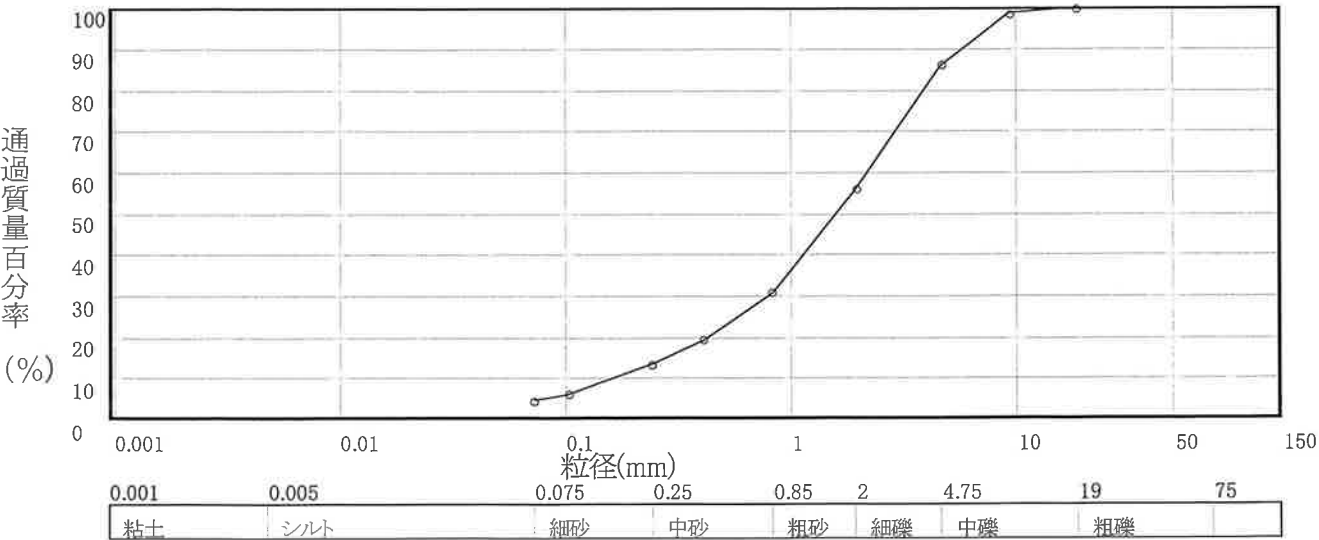
粒径加積曲線
