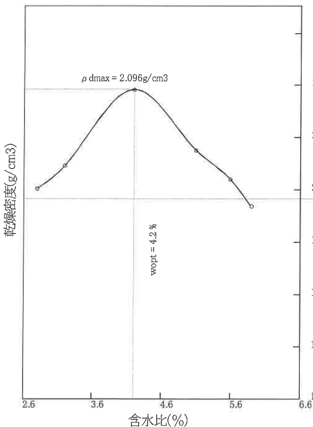
乾燥密度—含水比曲線
