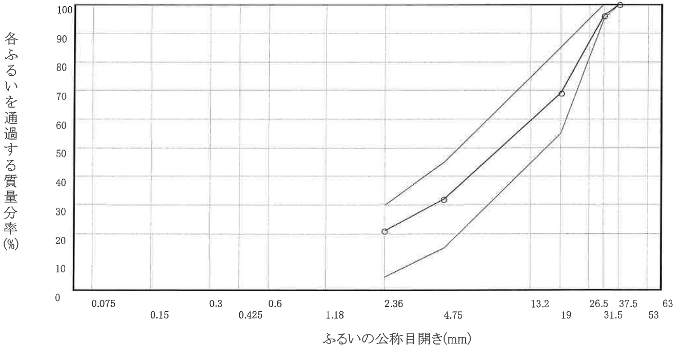
粒度曲線
